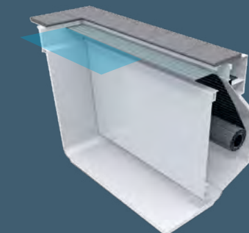
Die Nische verlängert das Becken um ca. 35 cm, verkürzt die Schwimmlänge um ca. 50 cm.
