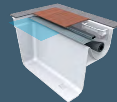
Der Rollladenschacht verlängert das Becken um 80 cm.
