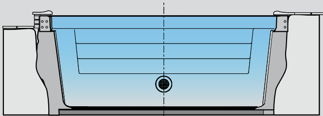
Einbau auf einer Bodenplatte. Variante für Freibäder.
